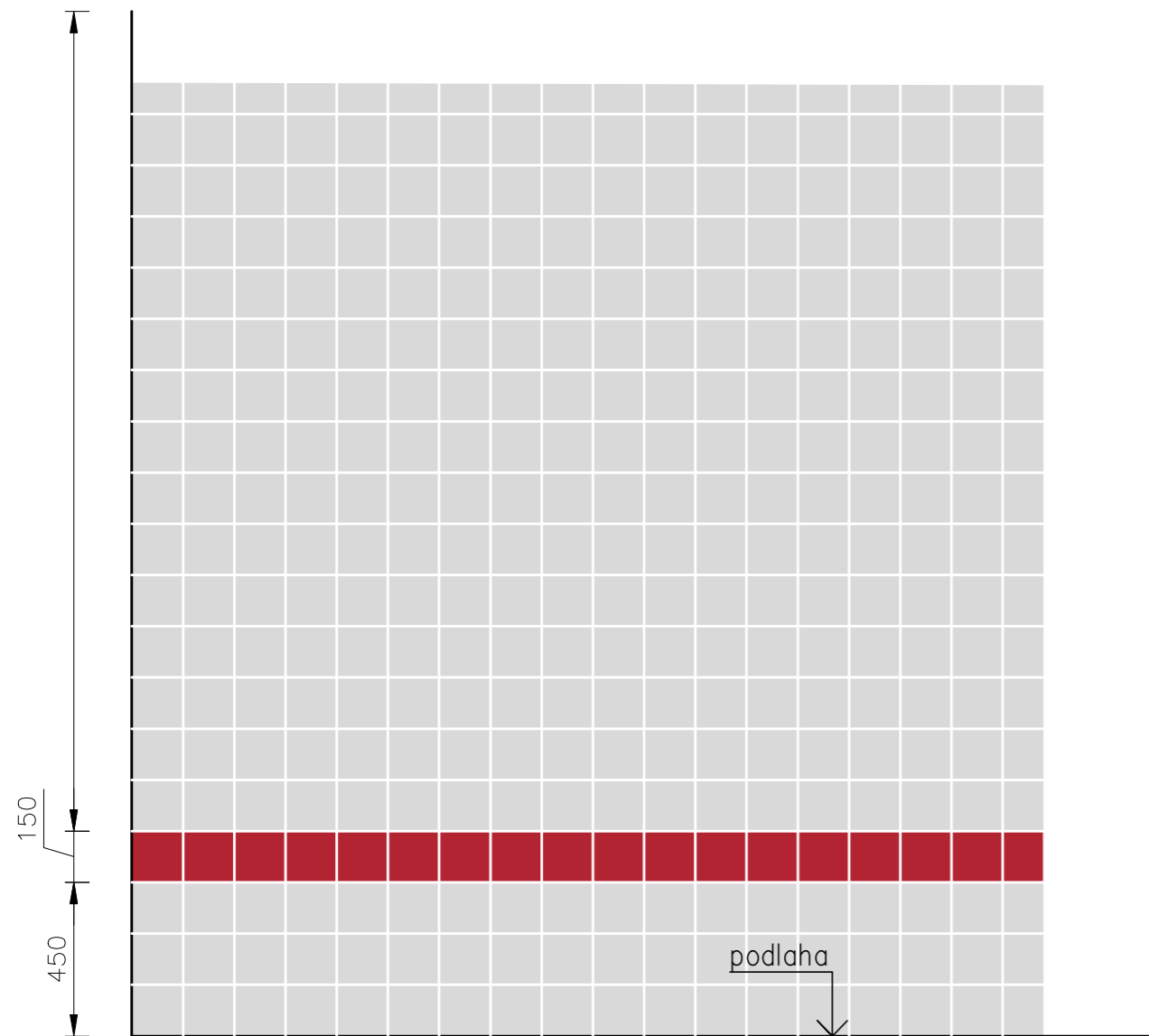
vzorová pokládka obkladu
